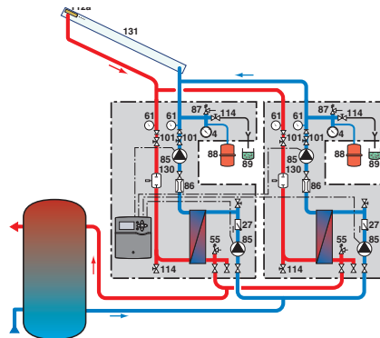
STS D 14-200 CME
