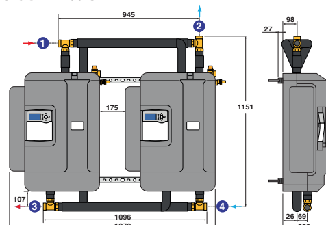
STS D 14-200 CME
