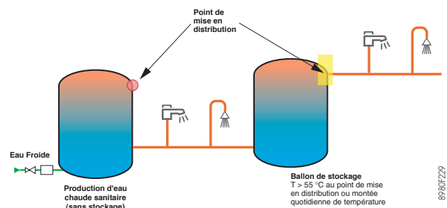
Exemple 2 : ballons de stockage présents en distribution
