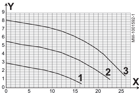
Fig.6 Pression disponible (circuit A)
