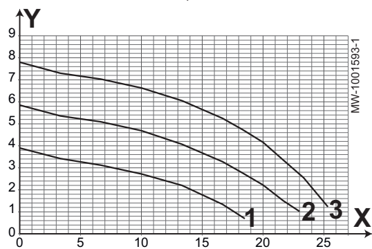
Fig.7 Pression disponible (circuit B avec des radiateurs)
