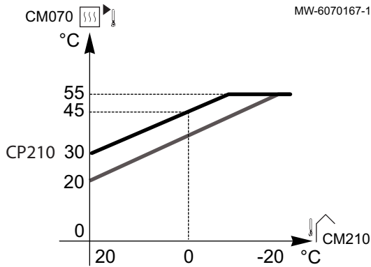
Fig.87 Courbe de chauffe avec pied de courbe
